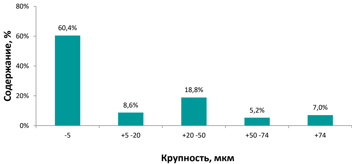
Рис. 4. Гранулометрический состав продукта измельчения
